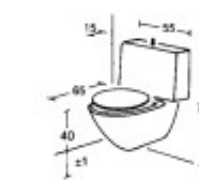
7 Wandspülklosett mit aufgesetztem Kasten
