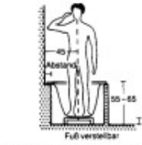
11 Nötiger Wandabstand zum Waschen, Einbauhöhen
