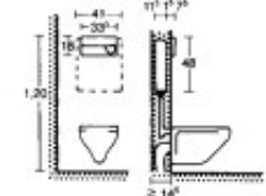
9 Tiefspülklosett mit eingebautem Spülkasten, 6 Liter Wasserverbrauch
