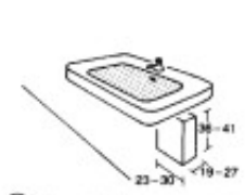
14 Untertisch-Warmwasserspeicher
