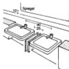
18 2 Waschbecken mit Handtuchhalter dazwischen
